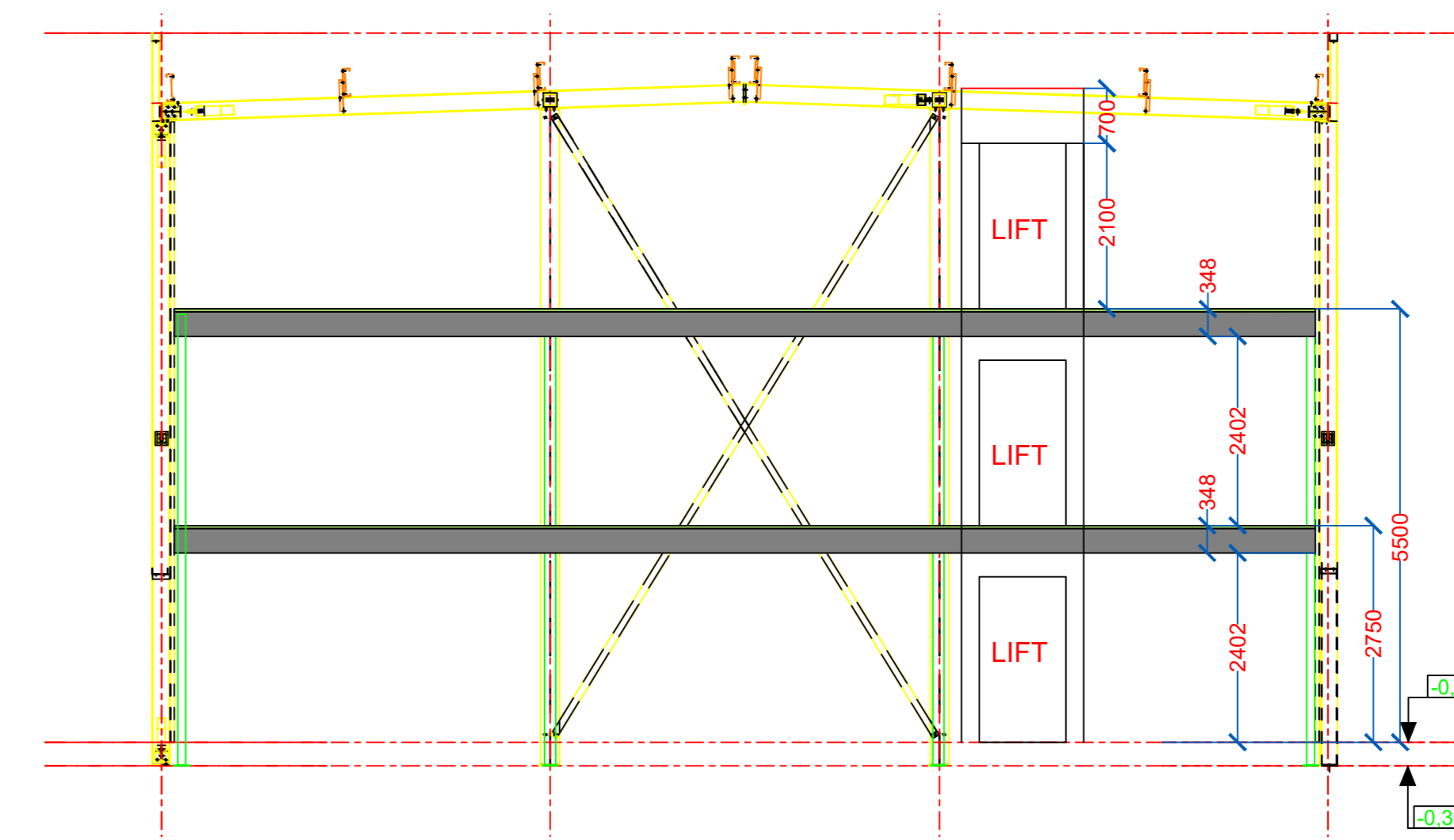
Coupe Schématique (sans échelle)
